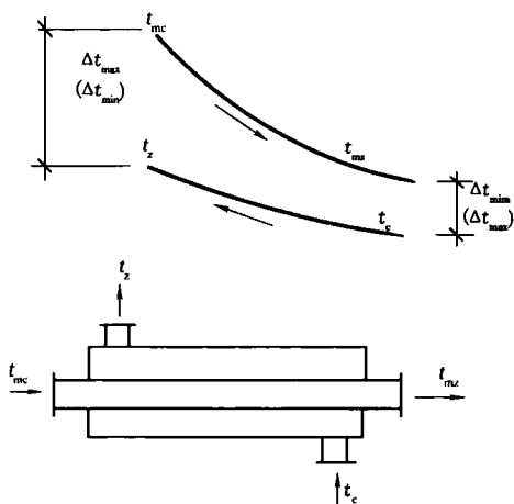
图6 快速水加热器水加热工况示意
